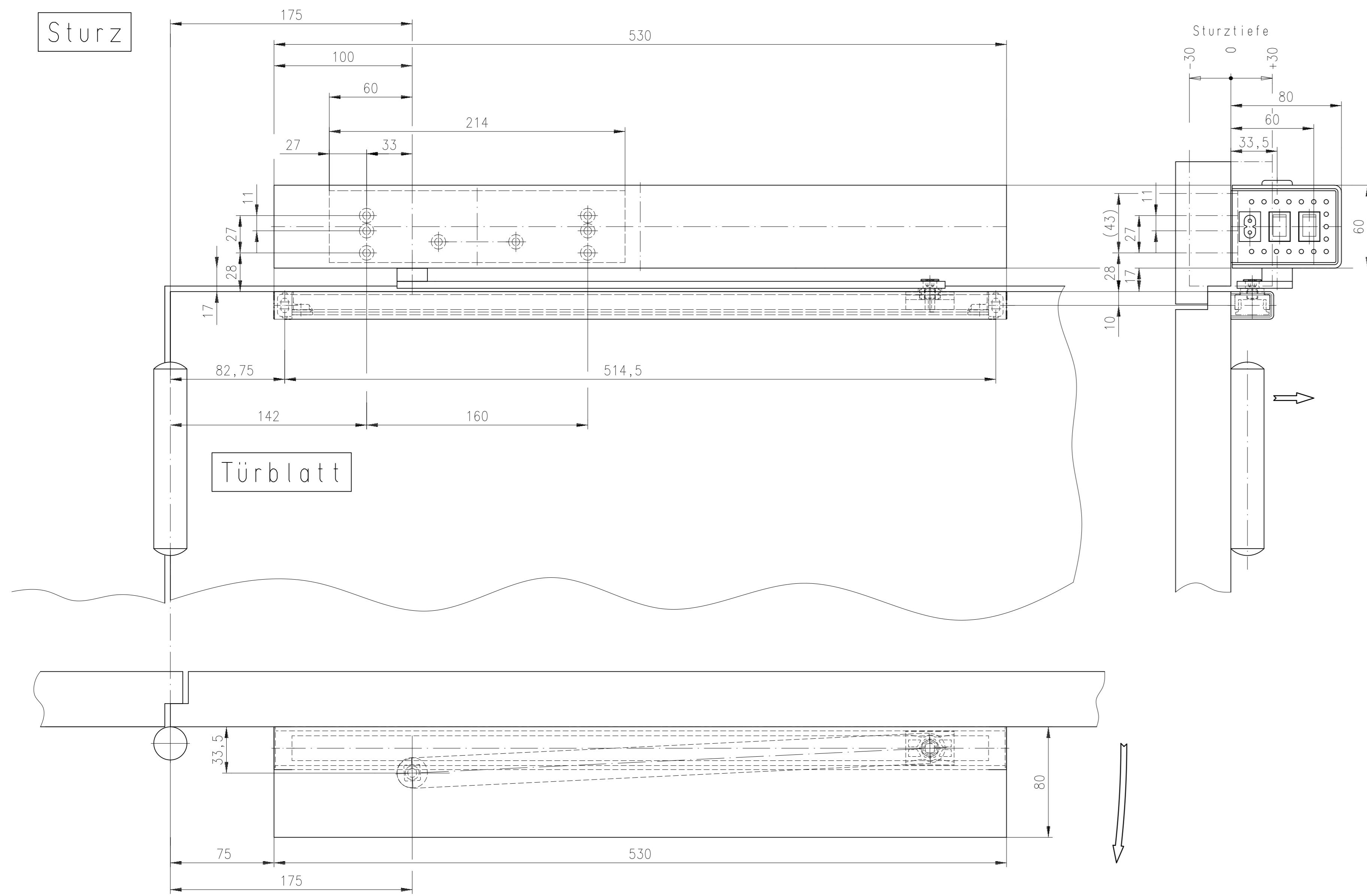
Sturzmontage Bandseite DIN links Sturzmontage Bandseite DIN rechts: spiegelbildlich
