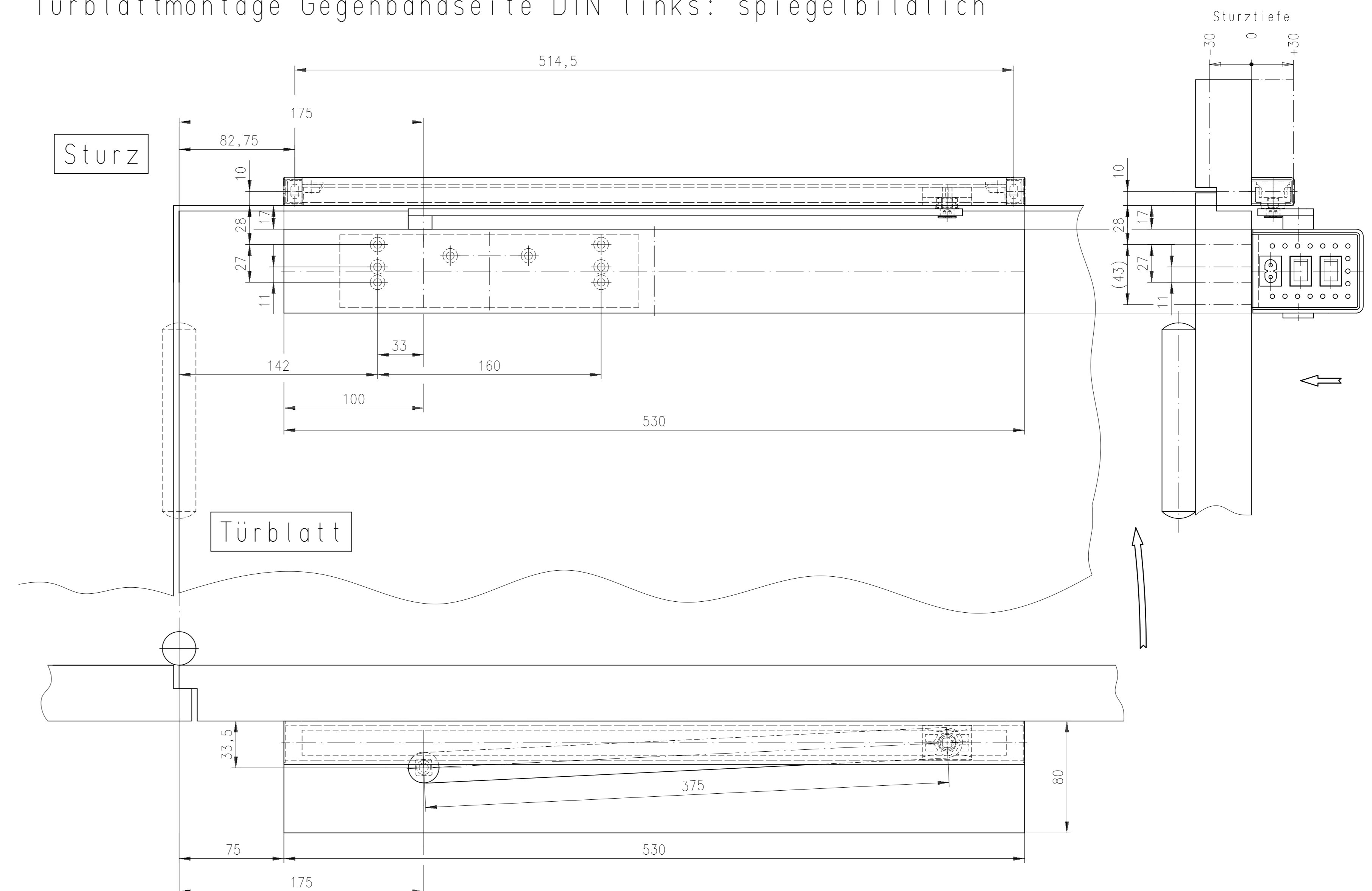
Türblattmontage Gegenbandseite DIN rechts Türblattmontage Gegenbandseite DIN links: spiegelbildlich
