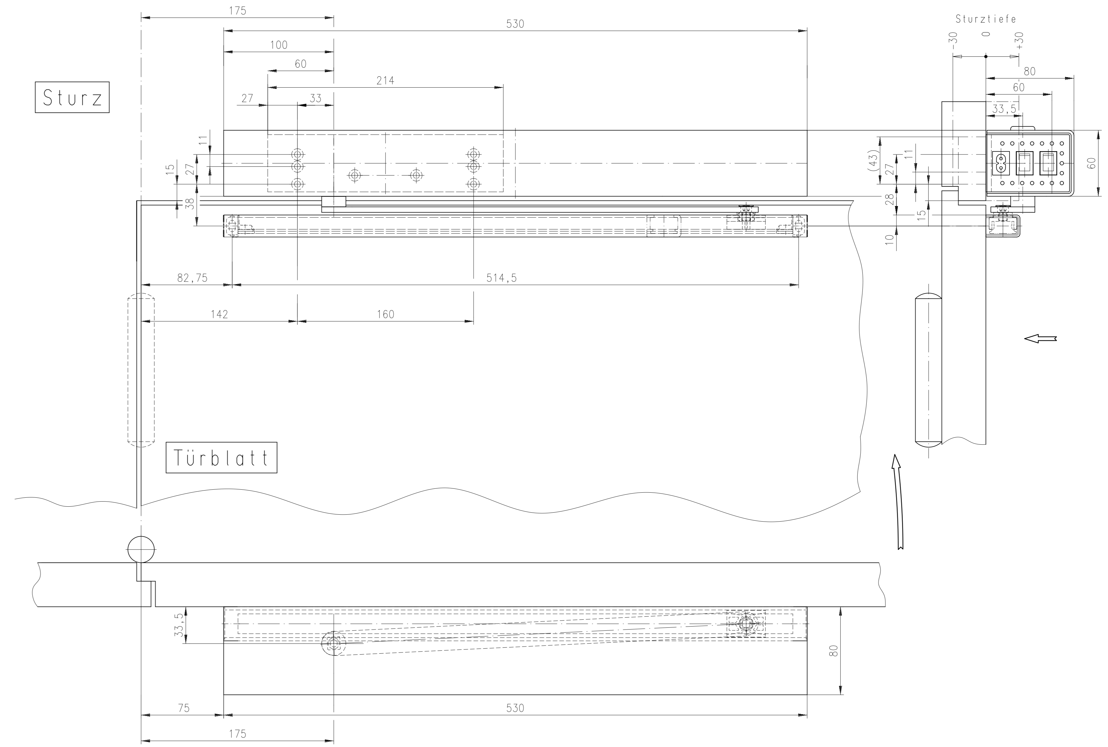
Sturzmontage Gegenbandseite DIN rechts Sturzmontage Gegenbandseite DIN links: spiegelbildlich
