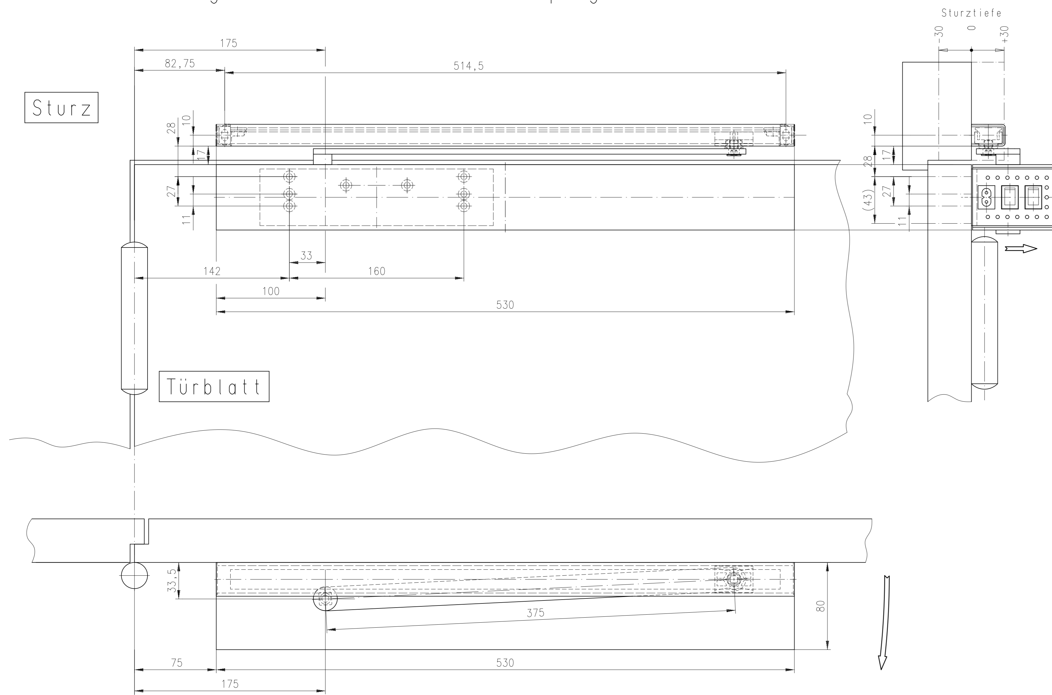
Türblattmontage Bandseite DIN links Türblattmontage Bandseite DIN rechts: spiegelbildlich
