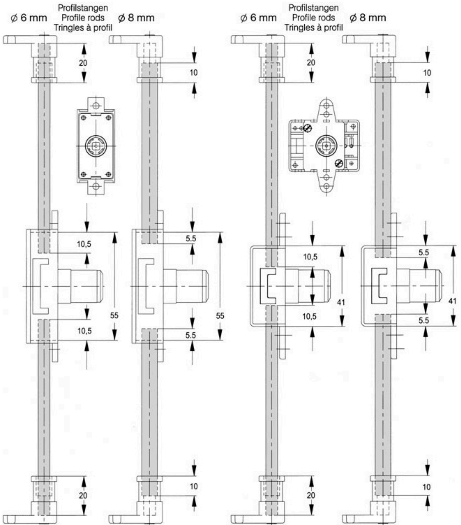
Drehstangenschlösser 8501; 8503 00002; 8505 15002; 8505 250002
